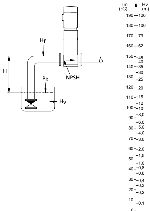
Рис. 25 Минимальный подпор - NPSH
