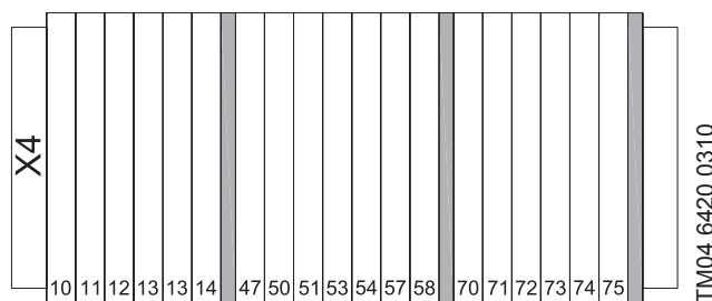
Рис. 10 Клеммная колодка
