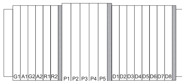
Рис. 11 Клеммная колодка
