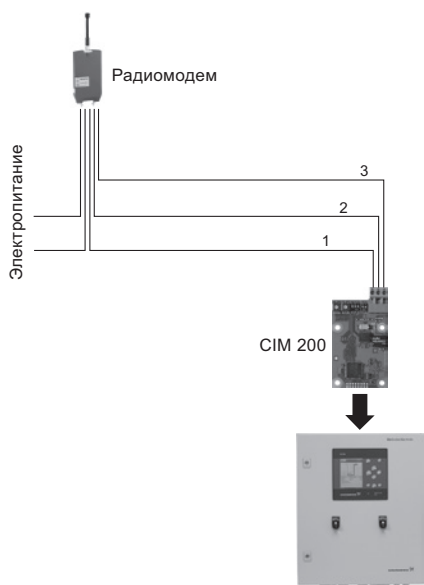
Рис. 23 Подключение радиомодема через Modbus RTU
