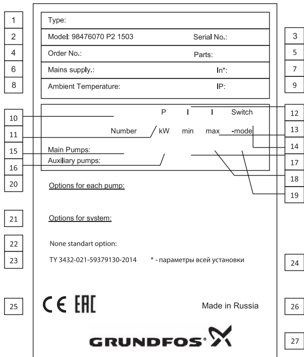
Рис. 2 Фирменная табличка
