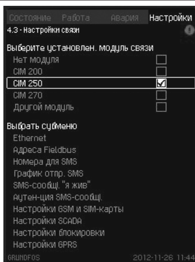
Рис. 21 Настройки связи
