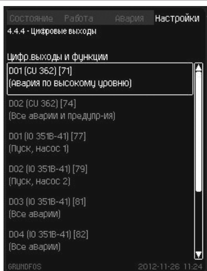
Рис. 33 Цифровые выходы
