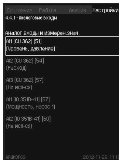
Рис. 27 Аналоговые входы
