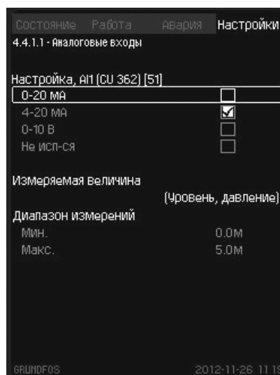
Рис. 28 Аналоговые входы
