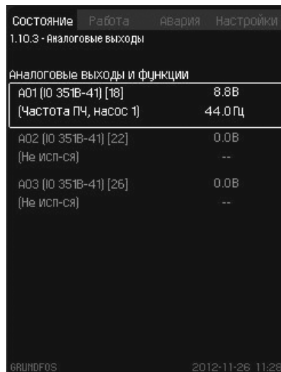
Рис. 40 Аналоговые выходы
