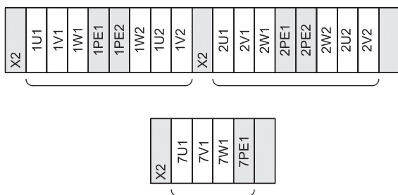
Рис. 8 Клеммные колодки
