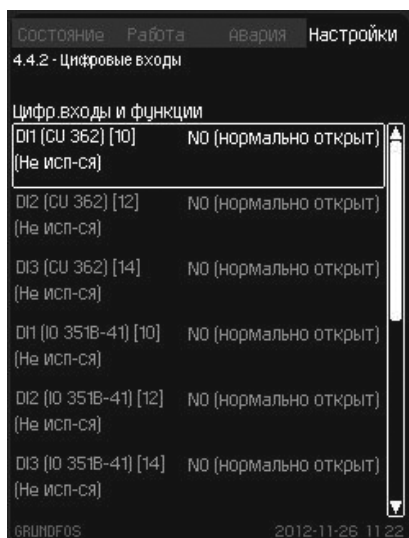
Рис. 30 Цифровые входы
