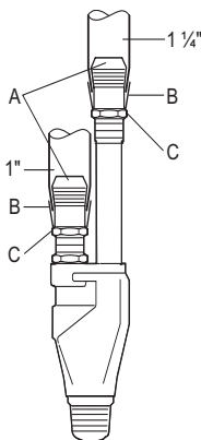
Obr. 3 Ejektor s plastovou přípojkou
